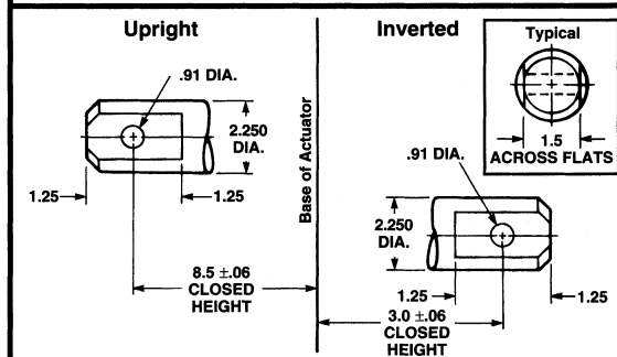
Clevis End
