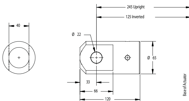
Clevis End G9010-11
