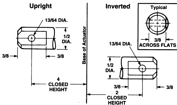
Clevis End
