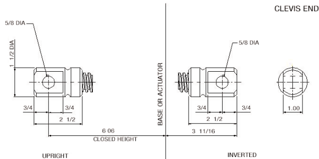
CLEVIS END
