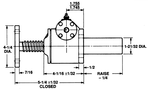
Upright: M-1802
