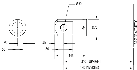
Clevis End G9020-11
